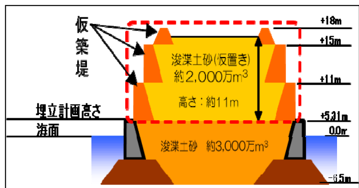
土砂処分場の断面図
