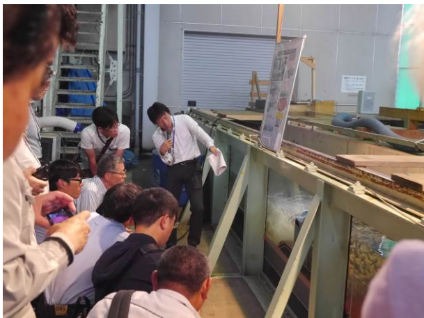
長水路水槽での防波堤効果実験
