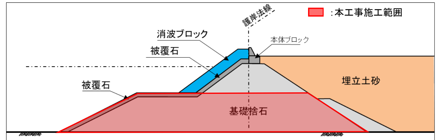
施工断面(イメージ図)
